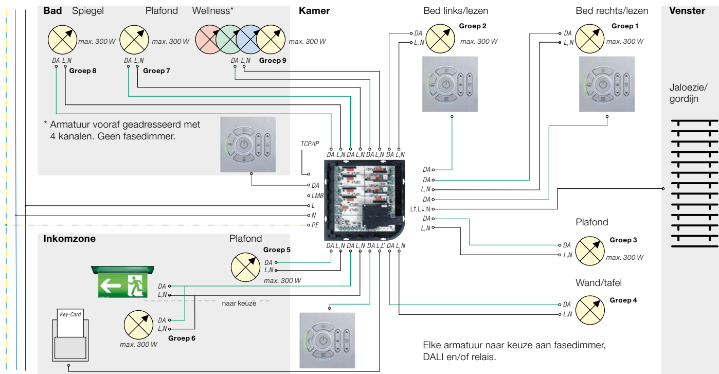
ZBOX Aansluitschema
