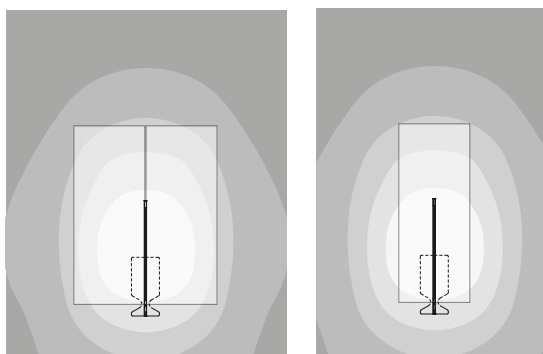
Espace de travail double ou simple : éclairage conforme à la norme EN 12464 pour un poste de travail avec un seul lampadaire
