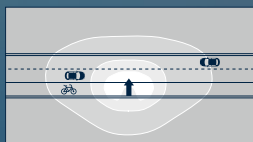
EXTENSIVE STREET (ES) CON DIFFUSORE
