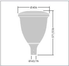
VOLUPTO Ø60 & Ø76
