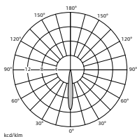
Stralingshoek 11°
